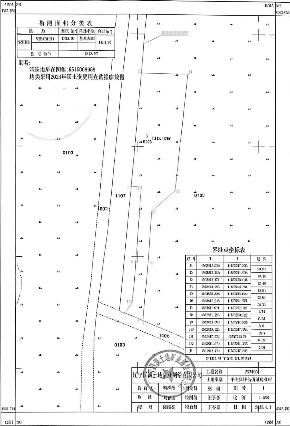
勘 测 正 界 图
